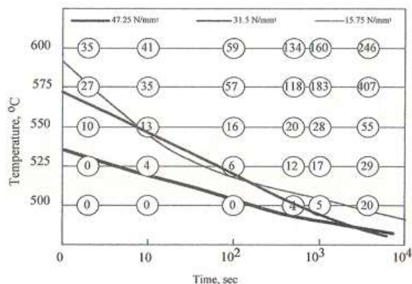
図3 加圧力を変えた時の金属間化合物層の厚さの変化 (沓名, M. Rathod) [2]
