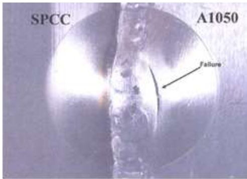
図8 SPCC鋼とアルミニウムの異材継手のエリクセン試験結果
