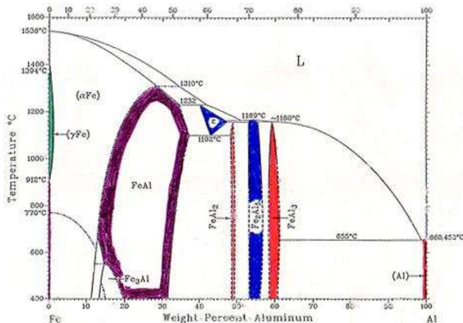
図1 Fe-Al系平衡状態図 (Hansen)
